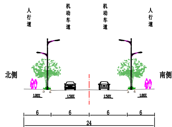
道路标准横断面图 惠安路 K0+399.247~K0+968.273
