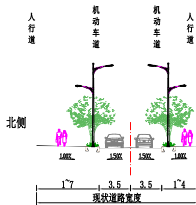
道路标准横断面图 龙溪南路
