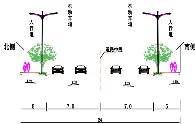
道路标准横断面图 乐高东路、临江北路
