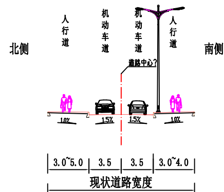
道路标准横断面图 祥新路
