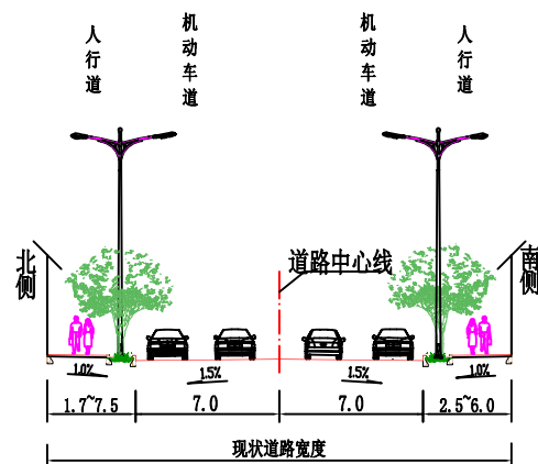
道路标准横断面图 观佛路
