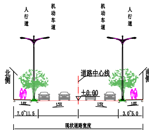
道路标准横断面图 福新路（观佛路至临江东路）
