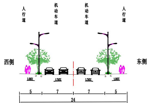
道路标准横断面图 桔荷路
