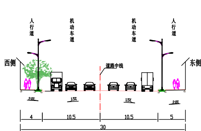
道路标准横断面图 碧水路
