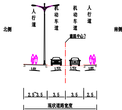
道路标准横断面图 规划道路（福新路至南新东路）
