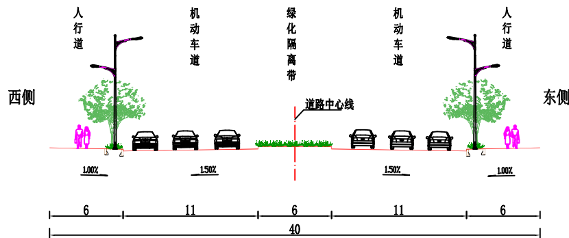
道路标准横断面图
