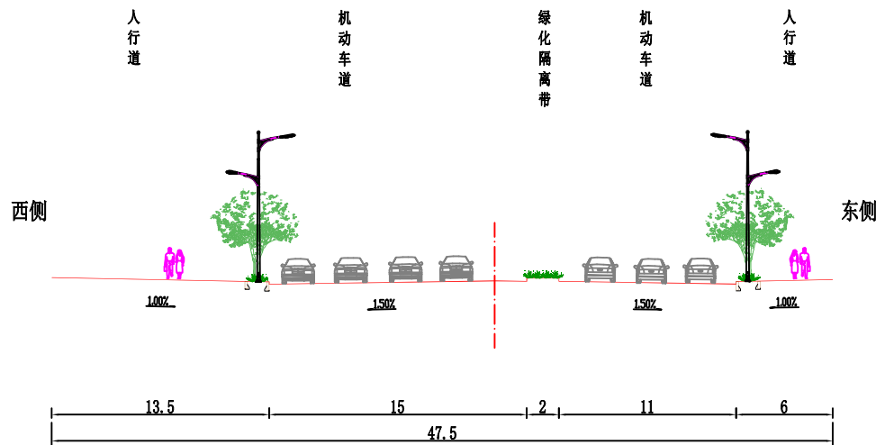
道路标准横断面图
