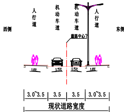
道路标准横断面图 规划道路I、II
