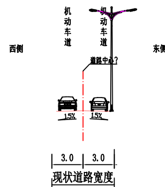
道路标准横断面图 规划道路III
