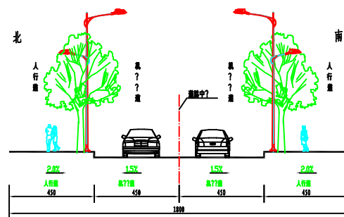
18m标准横断面图
