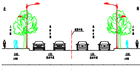
24m标准横断面图
