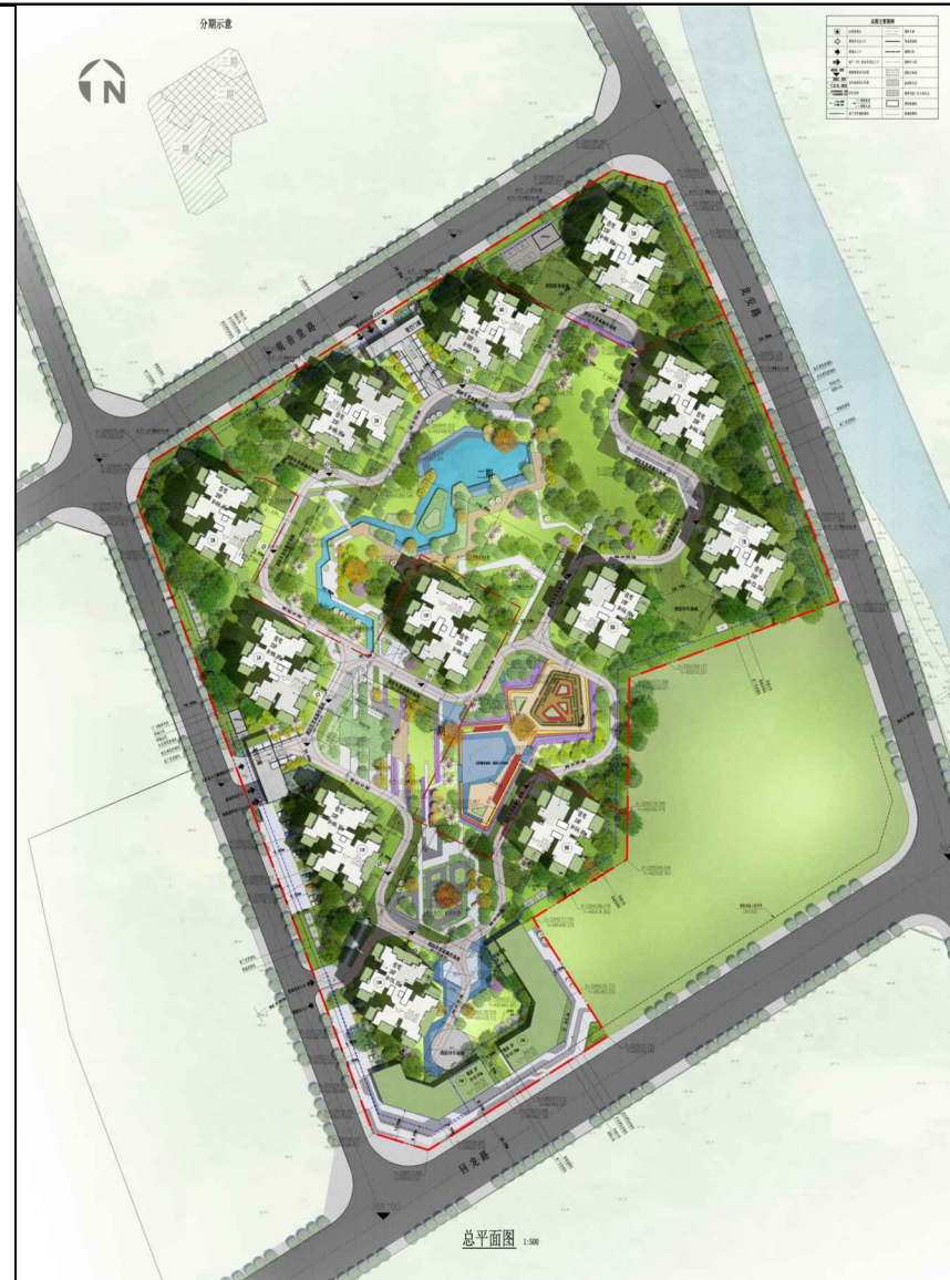
总平面布置图
