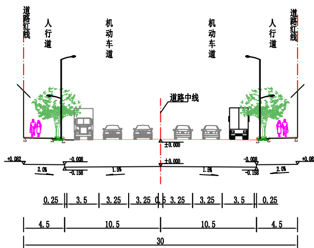
道路标准横断面图 (30m) 双林路(高港大道至碧水路段)
