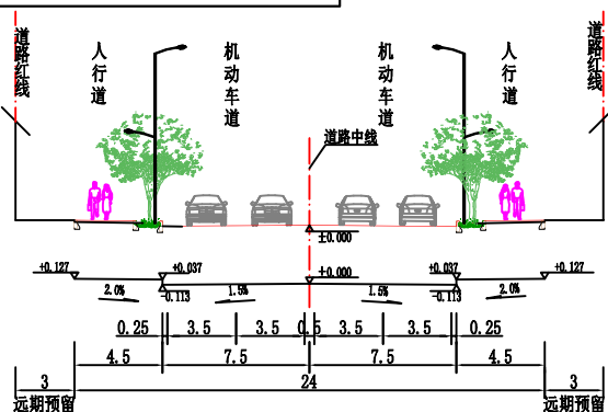
道路标准横断面图 (24m) 双林路(碧水路至桔荷路段)
