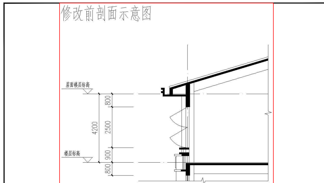
调整前剖面图
