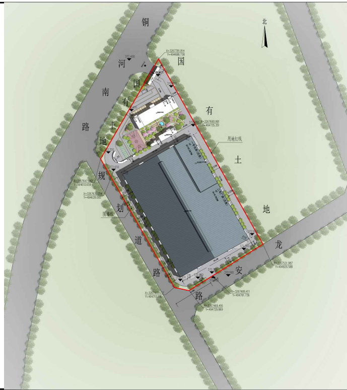
总平面布置图
